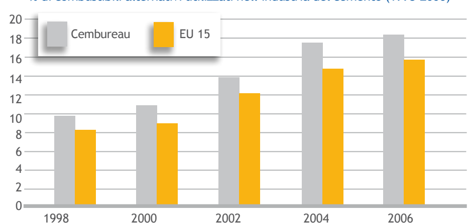
% di combustibili alternativi utilizzati nell'industria del cemento (1998-2006)
